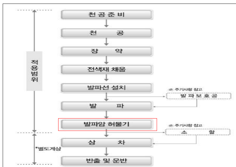
[그림 2] 암석 절취관련 공사 절차
